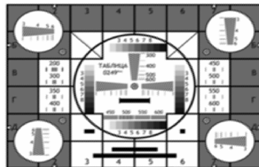
Сплайновая интерполяция
