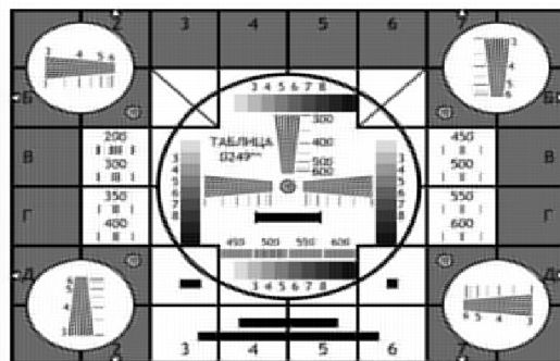
Метод IBP
