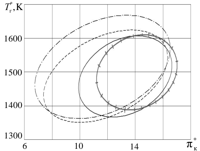
Рис. 2. Сопоставление областей оптимальных по критерию M_0 для различных дальностей полета:
