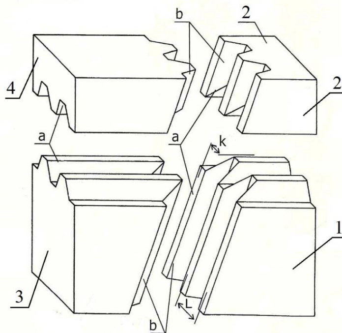
Рис. 4. Рабочие элементы оснастки для оппозитного формования
