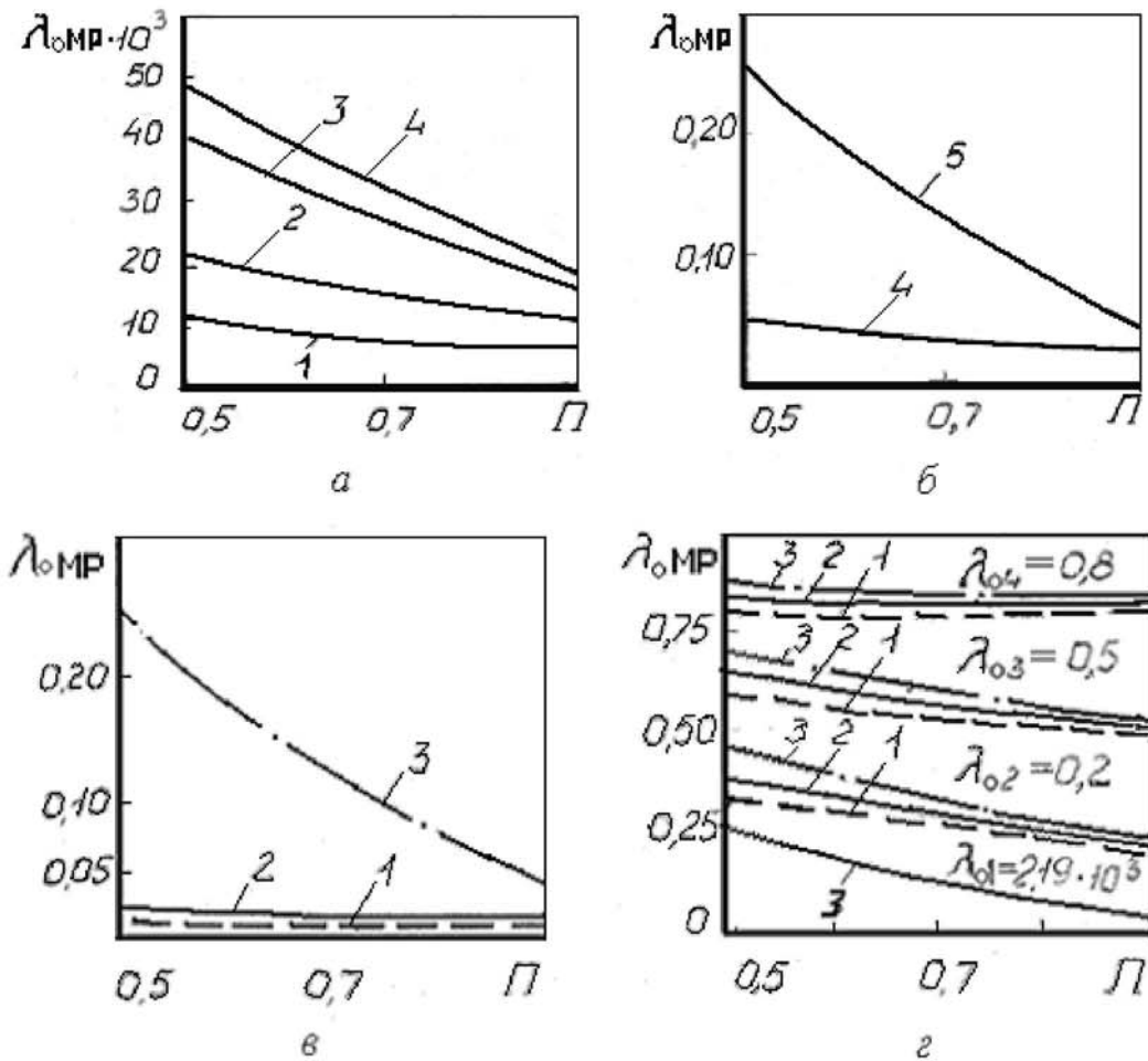
Рис. 2. Влияние параметров структуры на эффективную теплопроводность МР: а - \lambda_0 = 2,19 \cdot 10^3 ; 1 - n_n = 0 ; 2 - n_n = 0,5 ; 3 - n_n = 0,75 ; 4 - n_n = 0,8 ; б - \lambda_0 = 2,19 \cdot 10^3 ; 4 - n_n = 0,8 ; 5 - n_n = 1 ; в - \lambda_0 = 2,19 \cdot 10^3 ; 1 - n_n = 0 ; 2 - n_n = 0,5 ; 3 - n_n = 1 ; г - 1 - n_n = 0 ; 2 - n_n = 0,5 ; 3 - n_n = 1 при \lambda_{01} = 2,19 \cdot 10^3 ; \lambda_{02} = 0,2 ; \lambda_{03} = 0,5 ; \lambda_{04} = 0,8
