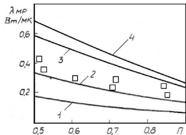
Рис. 1. Коэффициент эффективной теплопроводности МР:
