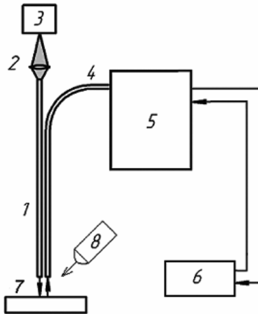
Рис. 2 - Экспериментальный стенд:
