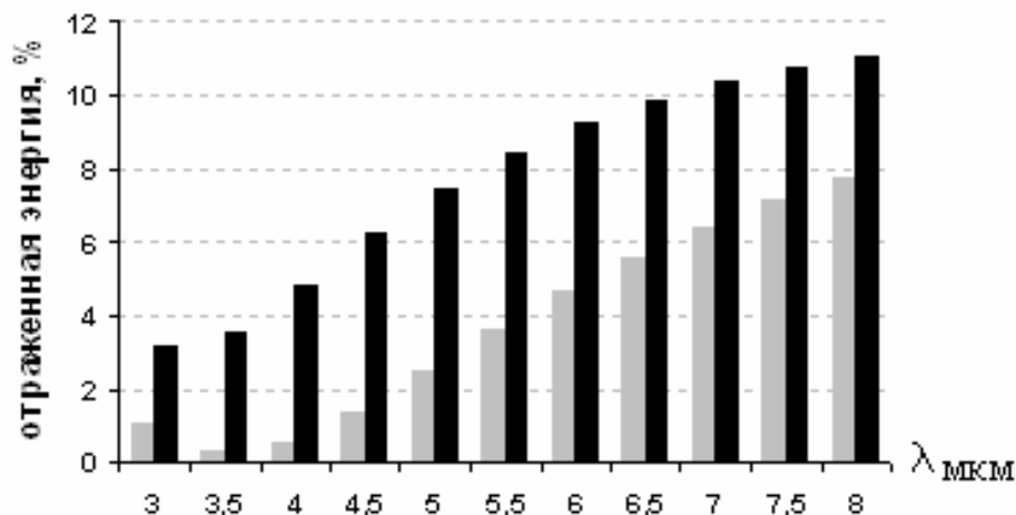
Рис. 2. Зависимость антиотражающего эффекта от типа волны (TE – серые столбики, TM – черные) и длины волны при использовании технологии плазмохимического травления матрицы штамповки
