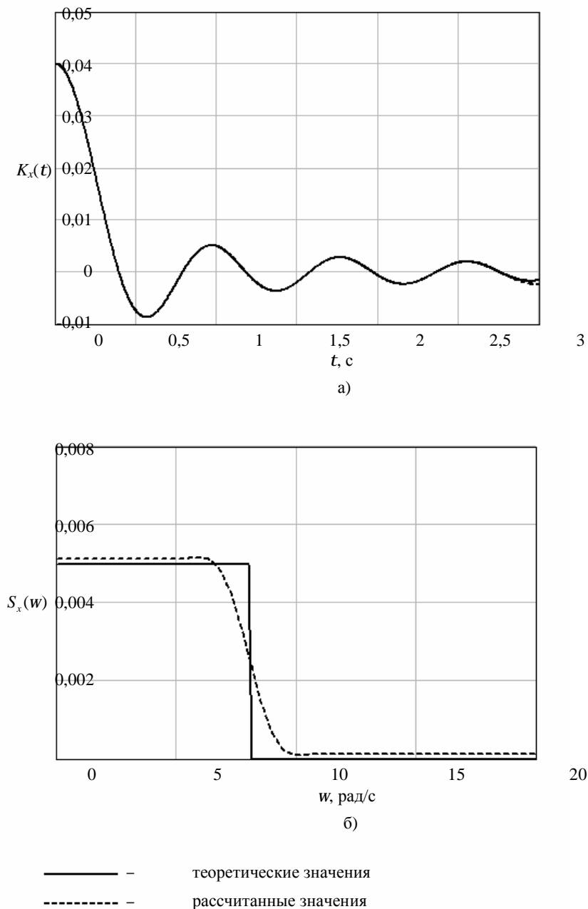
Рис. 1. Корреляционная функция (а) и спектральная плотность (б) узкополосного процесса №1 (число узлов q_g = q_d = 2 ; q_w = 8 )
