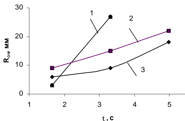
Рис. 8. Влияние турбулентности на динамику роста очага в зоне рециркуляции: горючее АСД-4; D_{КС} = 0,04 м ; 1 – без решетки ( e_0 = 5\% ), 2 – с решеткой на l_p = 0,02 м ( e_0 = 22\% ), 3 – с решеткой на l_p = 0,057 м ( e_0 = 12\% )
