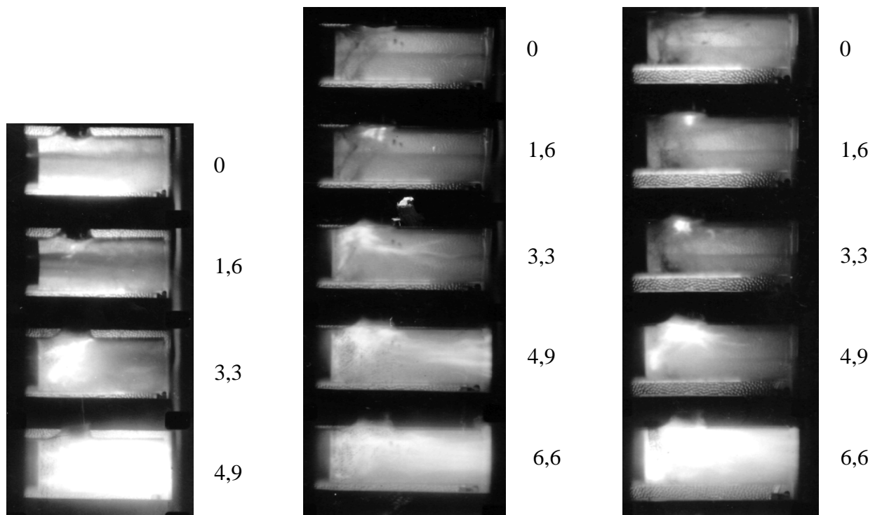
Рис. 7. Влияние начальной турбулентности e_0 на процесс развития очага в зоне рециркуляции; направление потока аэровзвеси слева на право: D_{КС} = 0,04\text{ м} ; горючее – АСД-4 ( d_{32} = 7,5\text{ мкм} ); а) – без решетки ( e_0 = 5\% ), б) – с решеткой на l_p = 0,02\text{ м} ( e_0 = 22\% ), в) – с решеткой на l_p = 0,057\text{ м} ( e_0 = 12\% ); цифры слева от снимков – время в мс, прошедшее от момента воспламенения
