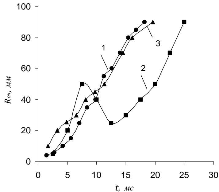
Рис. 9. Влияние начальной турбулентности воздуха e_0 на динамику роста очага при раздельной подаче компонентов аэровзвеси в камеру сгорания: D_{KC} = 0,09 м ; горючее – АСД-1 ( d_{32} = 17,5 мкм ); 1 – без решетки ( e_0 = 5\% ), 2 – с решеткой на l_p = 0,02 м ( e_0 = 22\% ), 3 – с решеткой на l_p = 0,057 м ( e_0 = 12\% )
