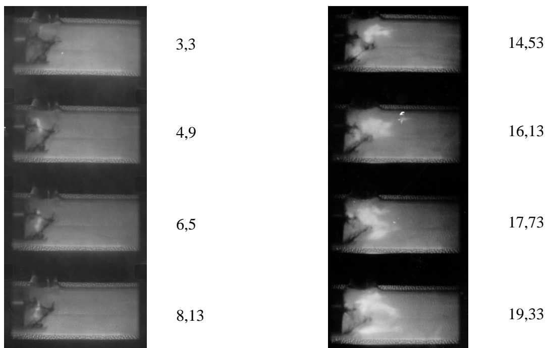
Рис. 5. Развитие очага в зоне рециркуляции камеры сгорания D_{КС} = 0,04 м : горючее – АСД-1 ( d_{32} = 17,5 \mu m ); направление потока аэрозвеси слева направо; параметры потока: U_0 = 50 м / с ; a = 1,1 ; T_0 = 293 K ; цифры справа от снимков – время в мс, прошедшее от момента воспламенения
