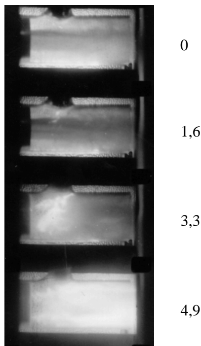
Рис. 6. Развитие очага горения в зоне рециркуляции: D_{КС} = 0,04 \text{ м} ; горючее – АСД-4 ( d_{32} = 7,5 \text{ мкм} ); направление потока аэрозвеси слева направо; параметры потока: U_0 = 50 \text{ м/с} ; a = 1,1 ; T_0 = 293 \text{ К} ; цифры справа от снимков – время в мс, прошедшее от момента воспламенения
