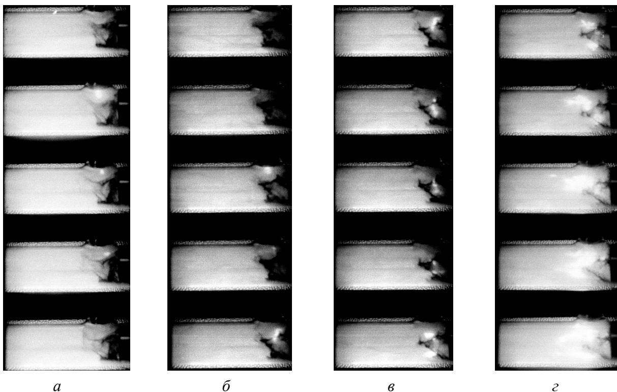
Рис. 1. Развитие начального очага в аэровзвеси частиц Al марки АСД-1 а – неудачное; б, в, г – успешное развитие; направление потока аэровзвеси справа налево; параметры потока: скорость на входе в камеру U_0 = 50 \text{ м / с} ; состав смеси \alpha = 1,1 ; температура аэровзвеси на входе T_0 = 293 \text{ К} ; скорость кино съемки – 600 кадр/с
