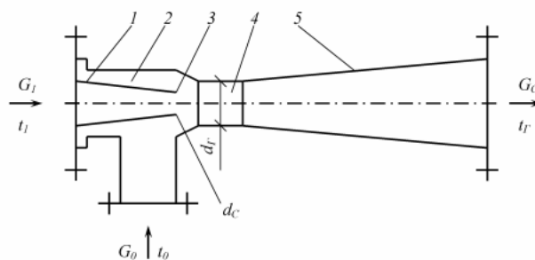
Рис. 1. Принципиальная схема водоструйного элеватора: 1 – сопло; 2 – камера всасывания; 3 – смесительный конус; 4 – горловина; 5 – диффузор
