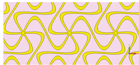
Рис. 4. Топология замедляющей системы печатной линзы Лüneберга: а - стандартном виде; б - увеличенном виде, соответствует изменению коэффициента замедления по закону
