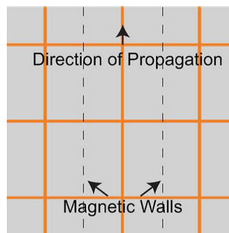
Рис. 1. Вид сверху на сетку из проводящих линий. Постоянная распространения радиоволн в сетке в \sqrt{2} раз больше, чем в отдельной линии
