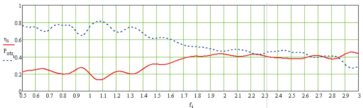
Рис. 9. КПД и доля мощности в балластах при нагрузке по 3 порта с каждой стороны от активного порта (всего 6) на балластные резисторы 50 Ом Fig. 9. Efficiency and power share in ballasts when loading 3 ports on each side of the active port (6 in total) on 50 Ohm ballast resistors
