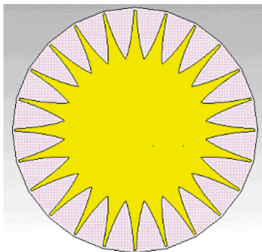
Рис. 3. Печатная линза Лüneберга: а - фрагмент стороны линзы с печатной замедляющей структурой (рис. 4); б - трансформаторы на основе НПЛ, запитывающие линзу Fig. 3. Printed Luneberg lens: a - a fragment of the lens side with a printed retarding structure (Fig. 4); b - NPL-based transformers that power the lens
