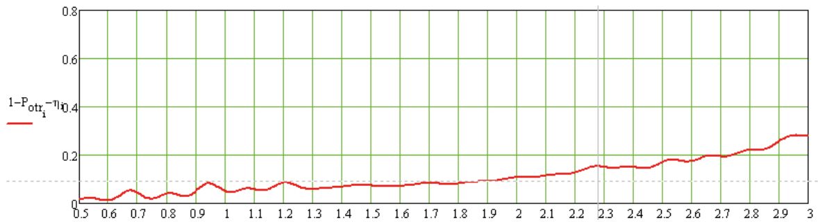
Рис. 7. Частотная зависимость омических и тепловых потерь в материалах линзы Fig. 7. Frequency dependence of ohmic and thermal losses in the lens materials
