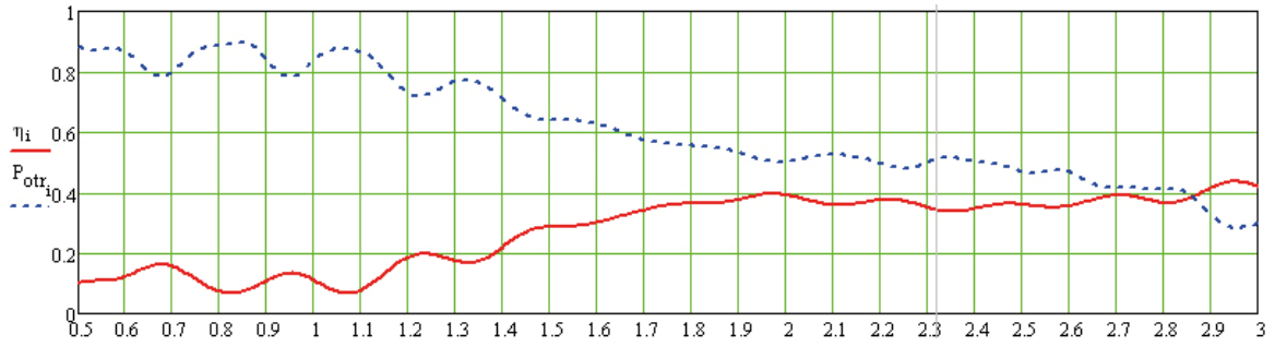
Рис. 6. Частотная зависимость КПД (сплошная линия) и мощность рассеянная в балластах (штриховая линия) Fig. 6. Frequency dependence of the efficiency (solid line) and the power scattered in the ballasts (dashed line)
