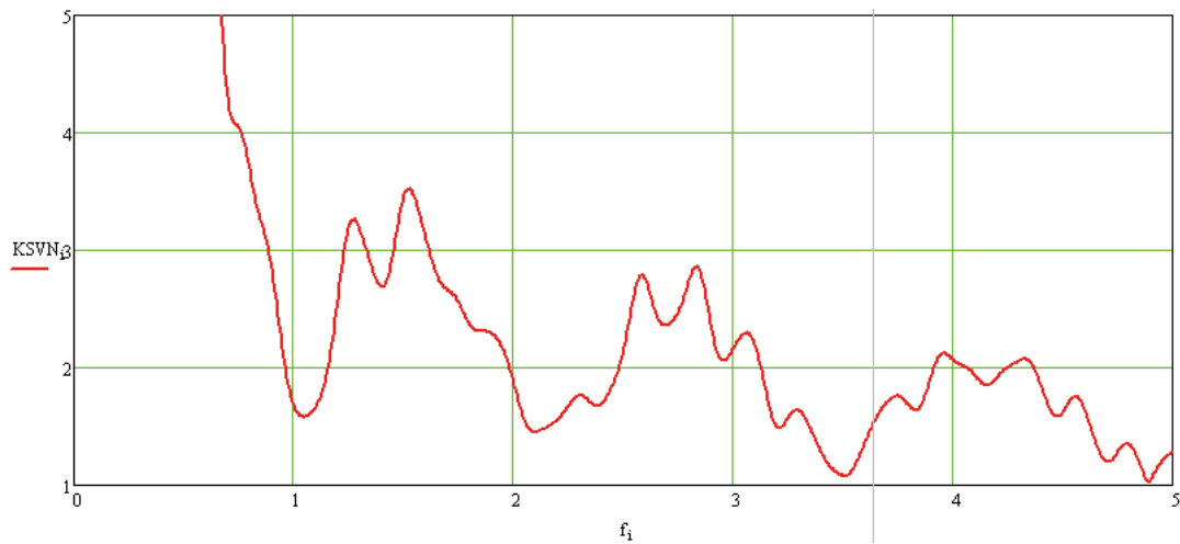
Рис. 8. Частотная зависимость КСВН Fig. 8. VSWR frequency dependence
