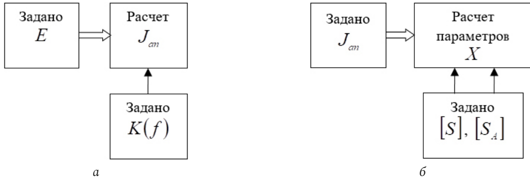
Рис. 2. Синтез параметров антенн для случая монохроматического сигнала. Этап 1. Синтез апертурного распределения (а), Этап 2. Расчет параметров антенны (б) Fig. 2. Synthesis of antenna parameters for the case of a monochromatic signal. Stage 1. Synthesis of aperture distribution (a), Stage 2. Calculation of antenna parameters (b)
