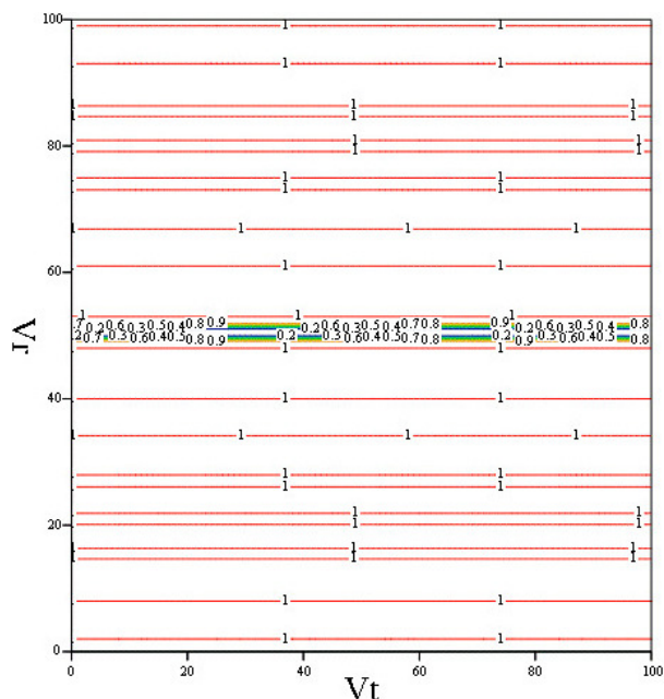
Рис. 5. p_{по} в зависимости от V_r \in [-300, 300] [м/с], V_r \in [-300, 300] [м/с] (на изображении индекс по осям меняется от 1 до 100), при наблюдении цели с ЭПР \sigma = 6 м 2 , базе интерферометра 2 м, пространственное разрешение 6 м для случая одновременного приема на две базы и использования режима автоматической фокусировки мобильных целей
