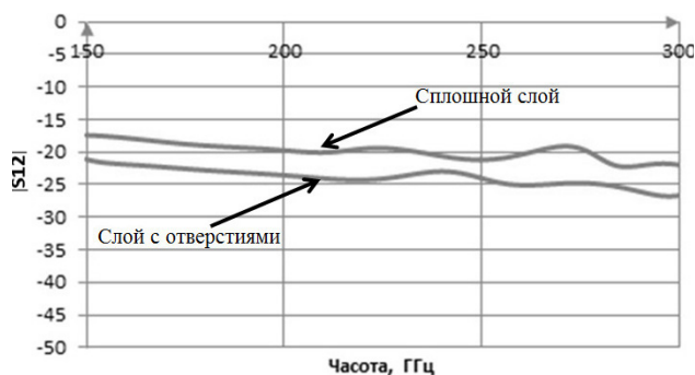
Рис. 16. Погонные потери (в дБ/мм) для сплошного слоя и слоя с отверстиями
