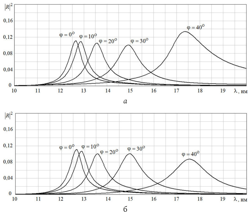
Рис. 5. Зависимости квадратов модулей коэффициентов отражения от длины волны (для углов падения плоской электромагнитной волны 0^\circ, 10^\circ, 20^\circ, 30^\circ, 40^\circ ) для структуры, состоящей из слоев пары сурьма/карбонат бора ( Sb / B_4C ): a – s -поляризация; б – p -поляризация Fig. 5. Dependences of the squares of the moduli of the reflection coefficients on the wavelength (for angles of incidence of a plane electromagnetic wave 0^\circ, 10^\circ, 20^\circ, 30^\circ, 40^\circ ) for a structure consisting of layers of an antimony/boron carbonate ( Sb / B_4C ) pair: a – s -polarization; b – p -polarization
