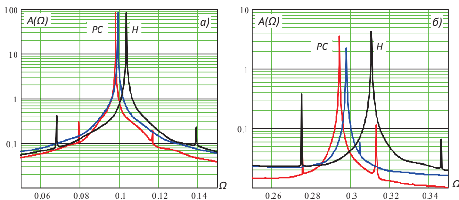
Рис. 2. Амплитудные спектры установившихся автоколебаний
