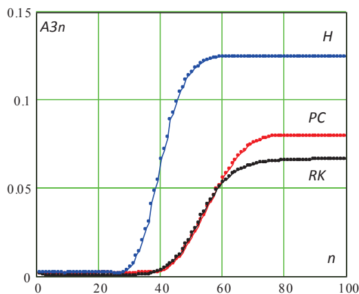
Рис. 3. Процесс установления амплитуды третьей гармоники
