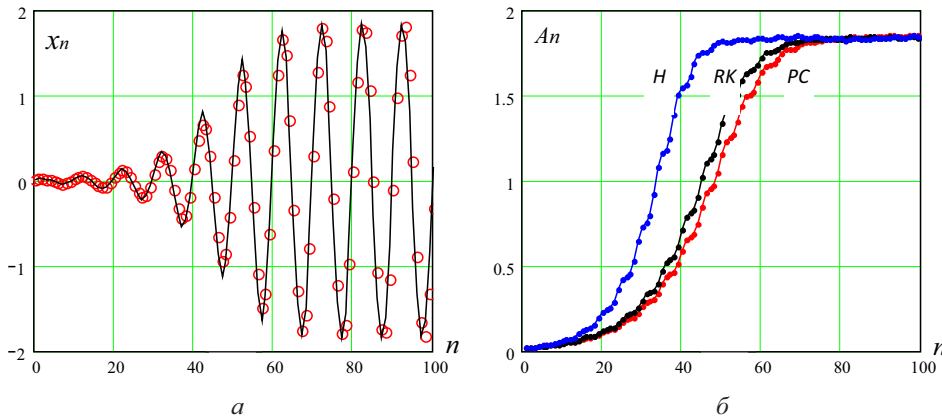
Рис. 1. Процесс установления автоколебаний
