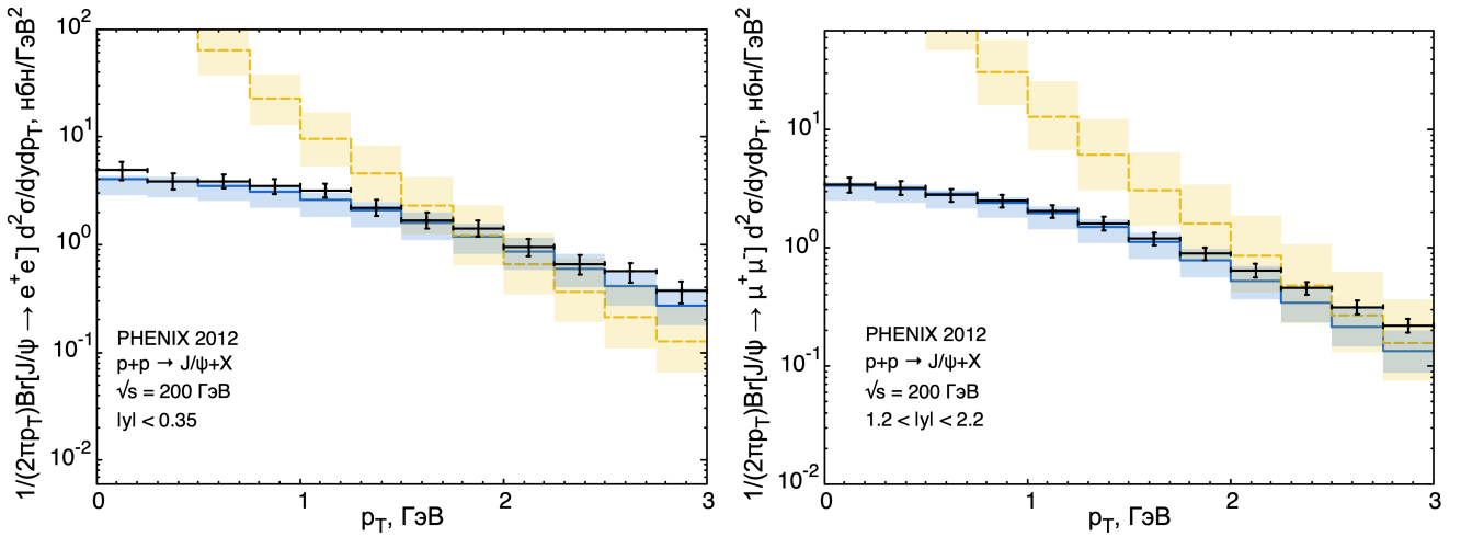
Рис. 3.7. Зависимость дифференциального сечения рождения J/\psi от поперечного импульса чармония p_T . Расчеты в КИМ (желтая штриховая линия) и ОПМ (синяя сплошная). Экспериментальные данные коллаборации PHENIX [27]
