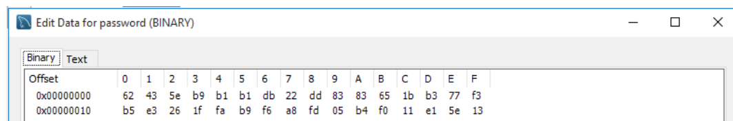
Рисунок 5. Хранение хеша паролей
